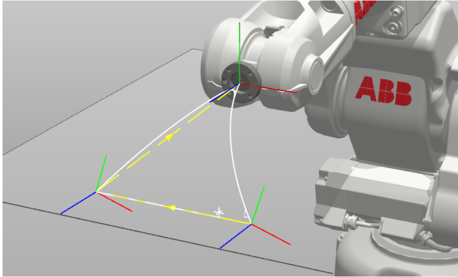
Figura 3: Robot con sus ternas en RobotStudio - movimiento horizontal
