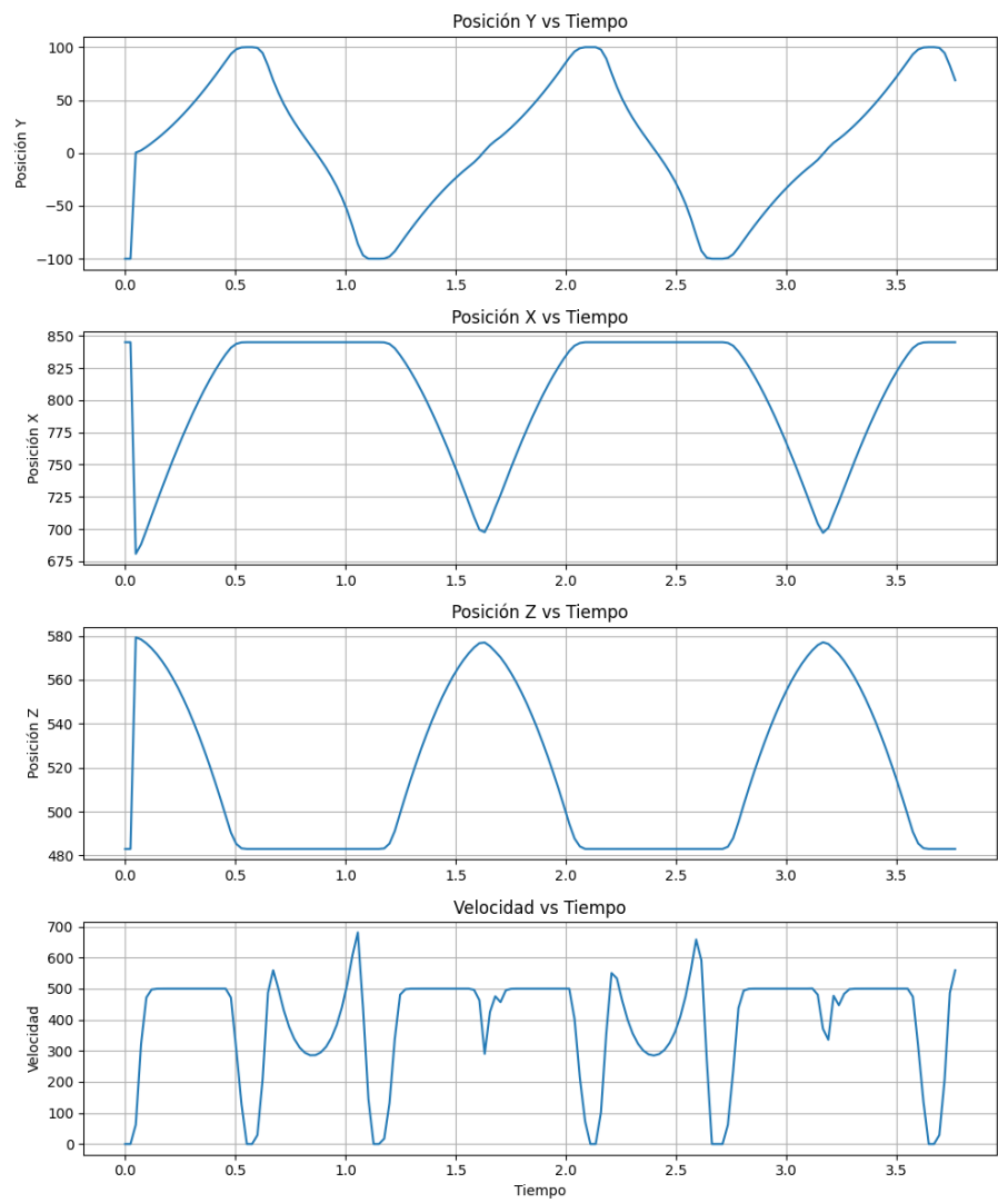
Figura 4: Posición y velocidad en función del tiempo - movimiento horizontal
