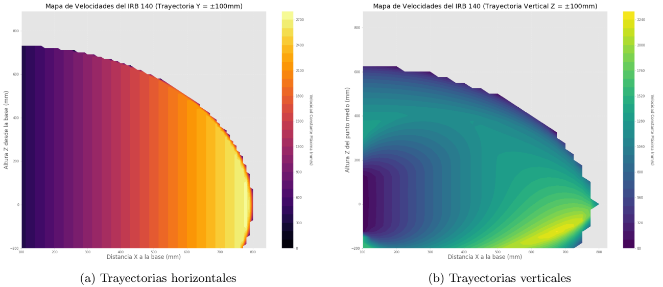
Figura 2: Mapas de calor de velocidades máximas para las trayectorias evaluadas
