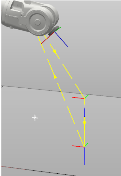
Figura 5: Robot con sus ternas en RobotStudio - movimiento vertical
